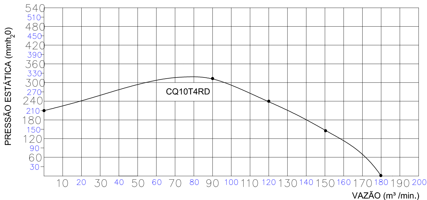
CURVA CARACTERÍSTICA (20°C/760 mm Hg)
