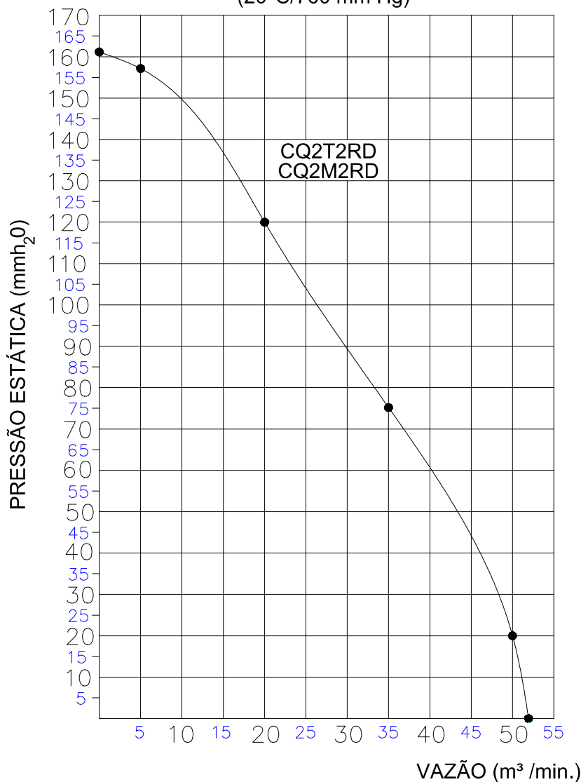
CURVA CARACTERÍSTICA (20°C/760 mm Hg)
