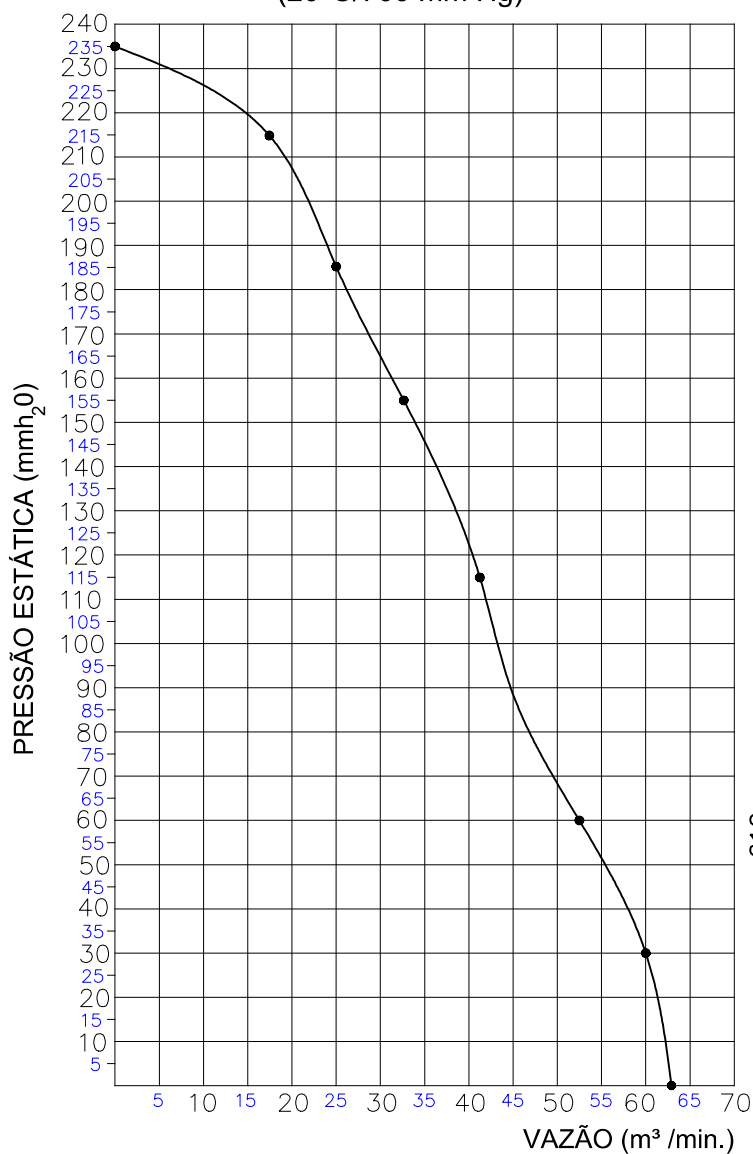
CURVA CARACTERÍSTICA (20°C/760 mm Hg)
