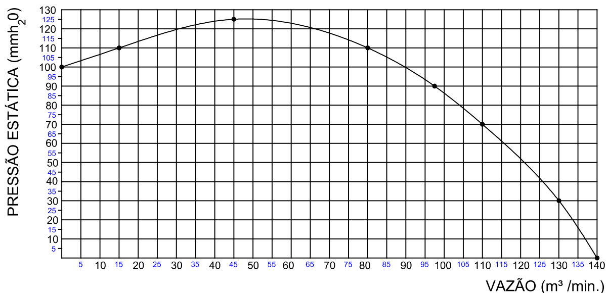
CURVA CARACTERÍSTICA (20°C/760 mm Hg)
