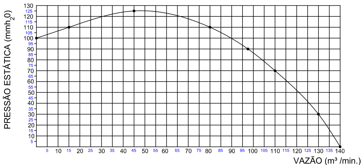
CURVA CARACTERÍSTICA (20°C/760 mm Hg)
