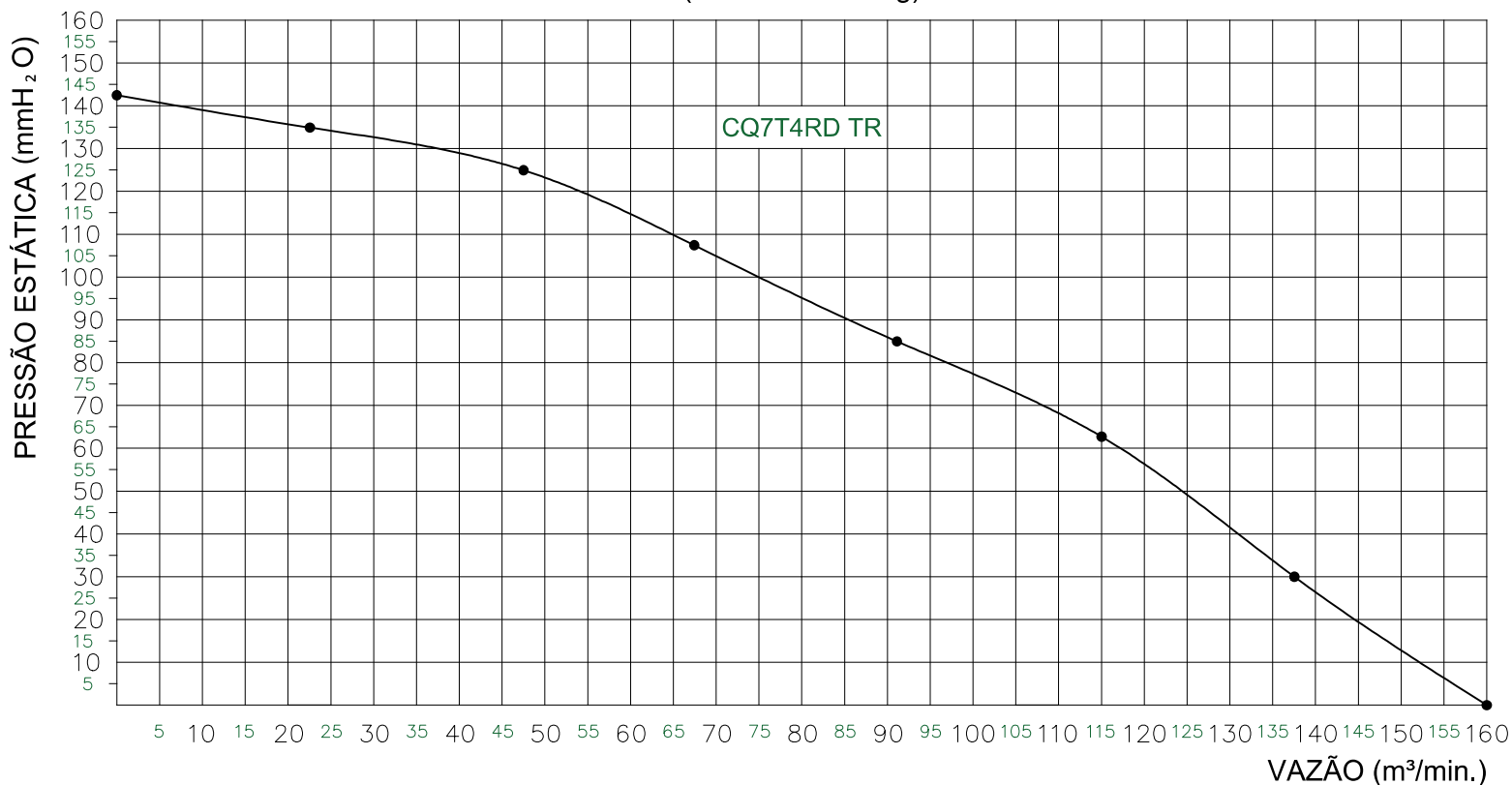
CURVA CARACTERÍSTICA ( 20^{\circ}\text{C}/760\text{ mm Hg} )
