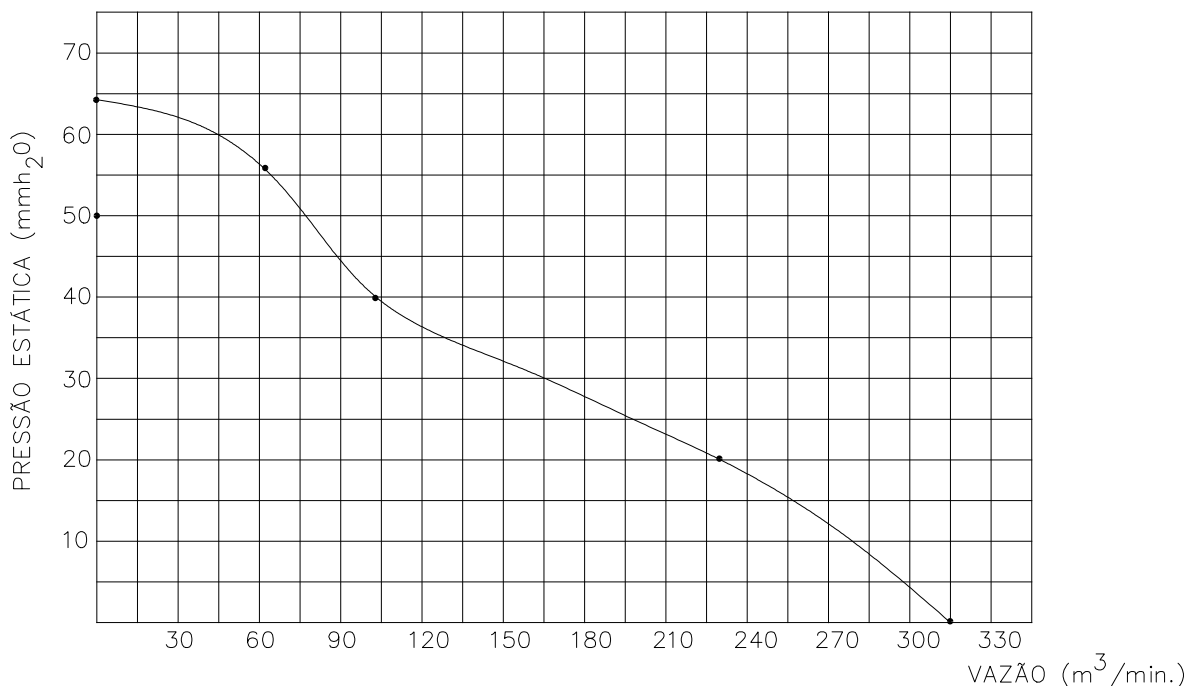
CURVA CARACTERÍSTICA (20°C/760 mm Hg)
