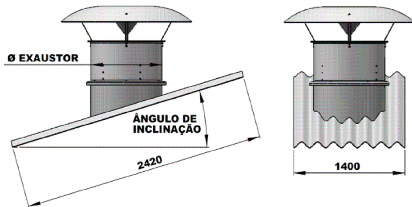
MEDIDAS E FORMATO DA TELHA ILUSTRATIVA
