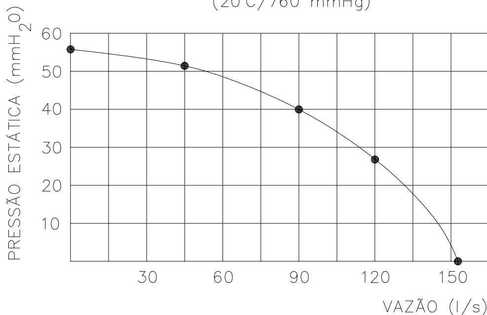
CURVA CARACTERÍSTICA ( 20^{\circ}\text{C}/760\text{ mmHg} )
