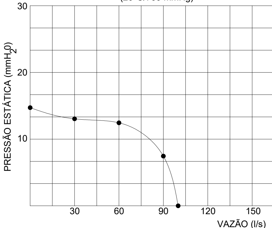
CURVA CARACTERÍSTICA (20°C/760 mmHg)
