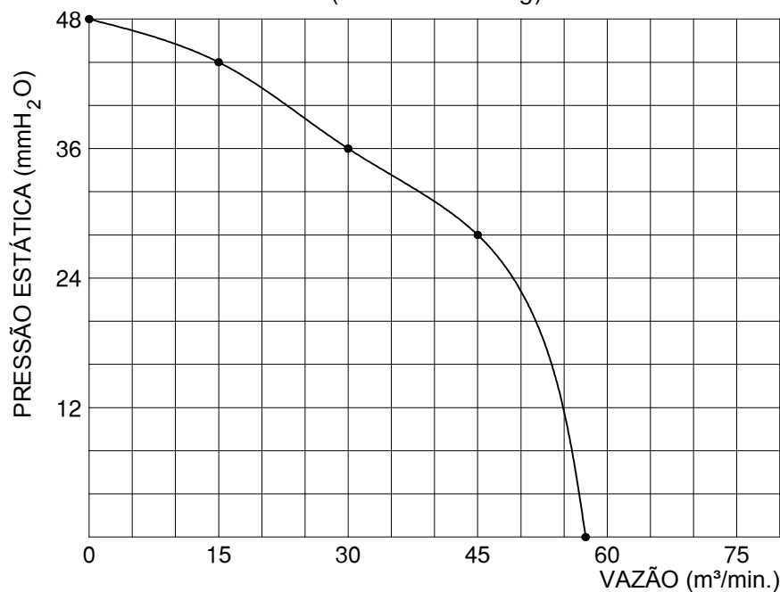
CURVA CARACTERÍSTICA (20°C/760 mm Hg)
